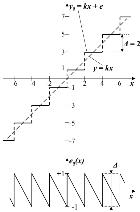
Fig. 3.18 Cuantizare și eroare de cuantizare (cuantizare uniformă)
