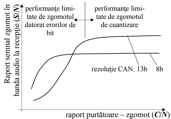
Fig. 3.23. Dependența raportului semnal zgomot de raportul purtătoare zgomot de canal în transmisiile cu MIC (reprezentare calitativă)
