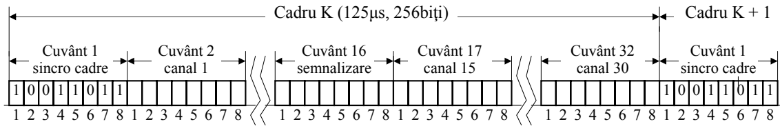
Fig. 3.18. Formatul de cadru în sistemul de multiplexare CCITT
