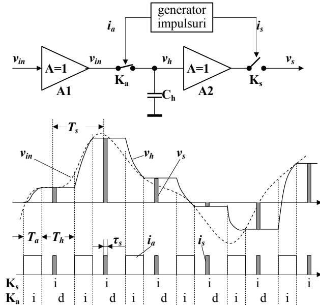
Fig. 3.4. Circuit de eșantionare și memorare (S & H). Schema bloc principală și diagramă de semnale
