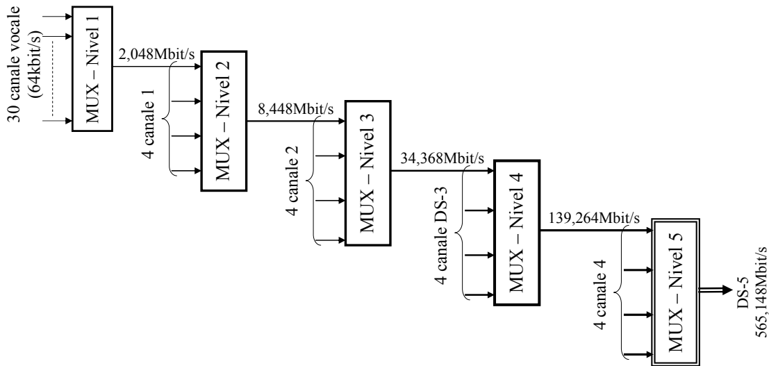
Fig. 3.17. Ierarhia CCITT de multiplexare în timp
