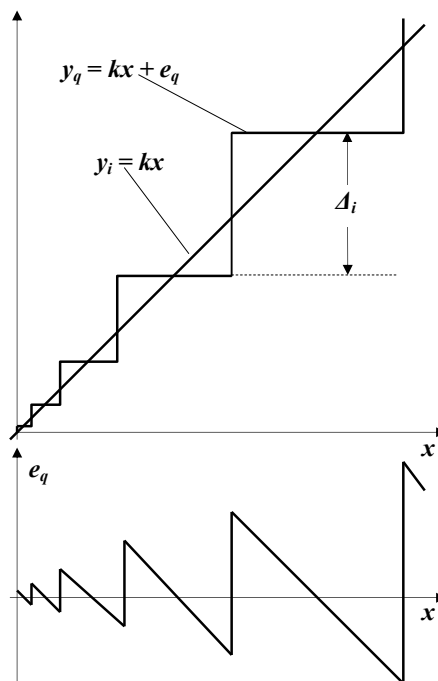
Fig. 3.19. Cuantizarea neuniformă și eroarea de cuantizare
