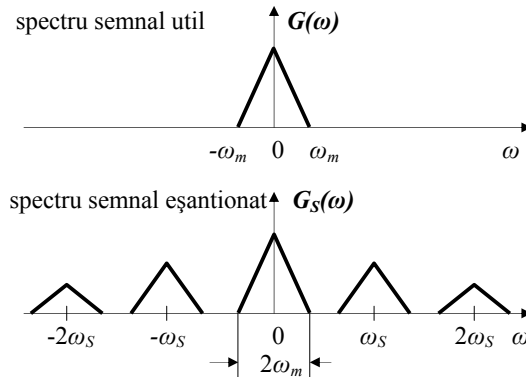
Fig. 3.3. Spectrul semnalului eșantionat
