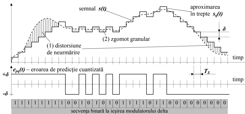
Fig. 3.27. Semnale în modulatorul delta (liniar, cu treaptă de cuantizare constantă)
