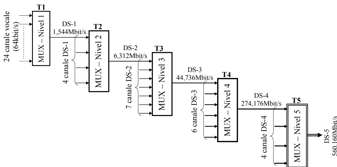
Fig. 3.17. Ierarhia de multiplexare în timp nord-americană
