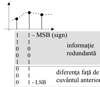
Fig. 3.24. Redundanța informației la codarea eșantioanelor
